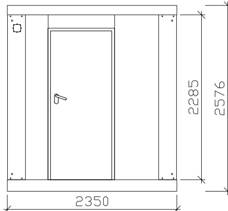
ALZADO LATERAL IZDO
